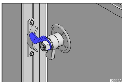
Obr. 15: Záchytné zařízení
