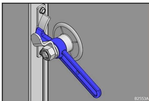
Obr. 16: Jazýček zarážky s vnitřní klikou
