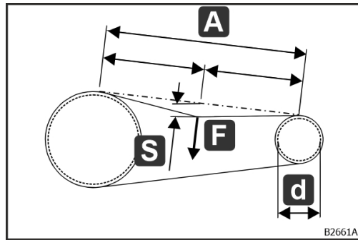
Obr. 22: Napnutie remeňa pri ventilátore so špirálovou skriňou
