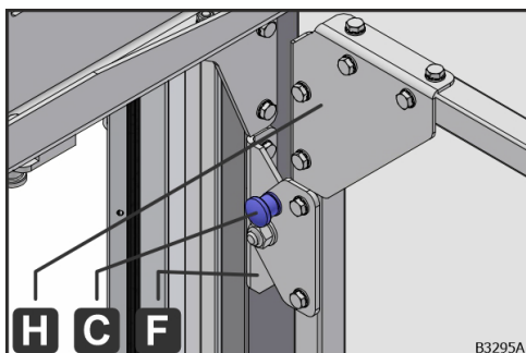
Obr. 77: Minirastre C-M10 (C) v závesných uholníkoch hore (F)
