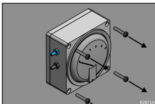
Obr. 145: Odstránenie skrutiek
