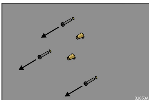
Obr. 128: Odstránenie skrutiek
