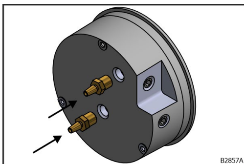
Obr. 132: Zaskrutkovanie hadicových objímok
