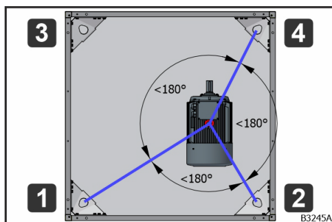
Obr. 85: Správne použitie rohových uzlov 1,2,3
