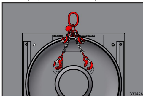
Obr. 32: Zavesenie viazacích reťazí pri dvoch viazacích okách
