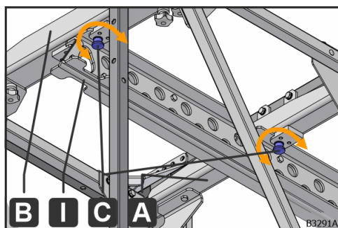
Obr. 71: Zaistenie nosného ramena s minirastrami
