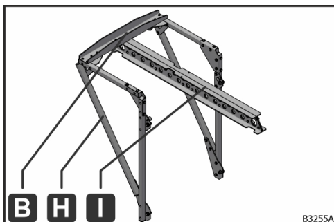
Obr. 55: Diely, ktoré sa namontujú na stavbe
