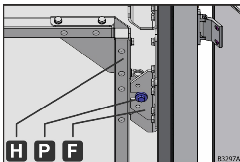
Obr. 110: Centrovacie čapy (P) v závesných uholníkoch hore (F)
