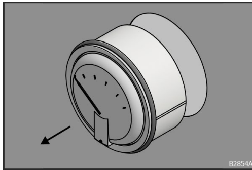
Obr. 129: Odobratie ručičkového manometra
