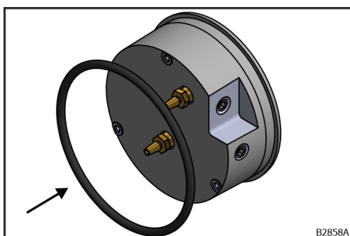
Obr. 133: Natiahnutie O-krúžka
