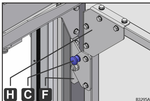
Obr. 112: Minirastre C-M10 (C) v závesných uholníkoch hore (F)
