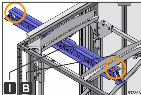
Obr. 66: Otvor v nosnom ramene (I)
