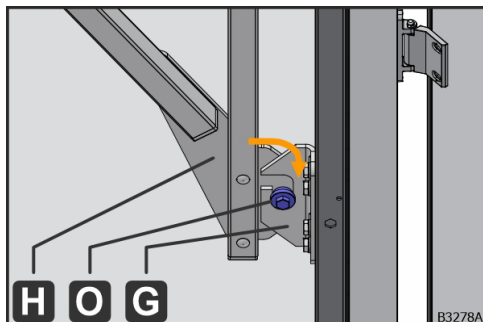
Obr. 59: Zavedenie centrovacieho čapu dole do drážky
