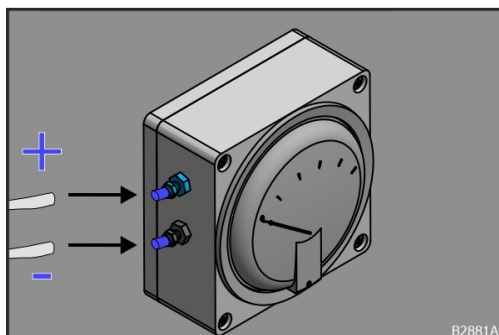
Obr. 159: Nasunutie hadíc merača tlaku
