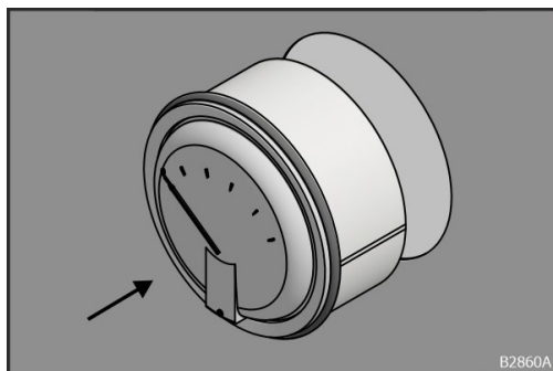
Obr. 135: Vloženie ručičkového manometra
