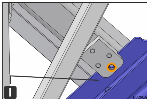
Obr. 70: Polohovanie nosného ramena pre zaistenie s minirastrami
