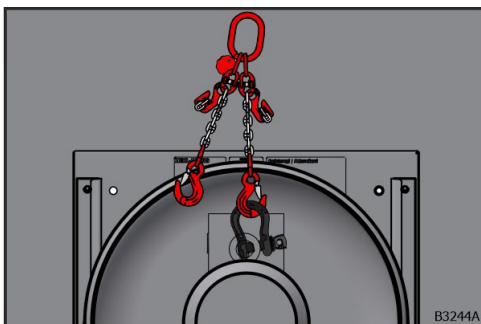
Obr. 84: Zavesenie viazacích reťazí pri jednom viazacom oku
