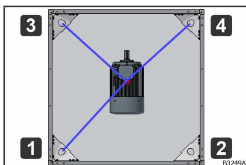
Obr. 40: Bremo v strede opláštenia s pákovým reťazovým kladkostrojom v rohových uzloch 4
