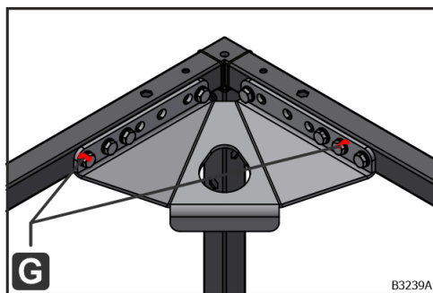
Obr. 31: G – Zaisťovací lak na skrutky
