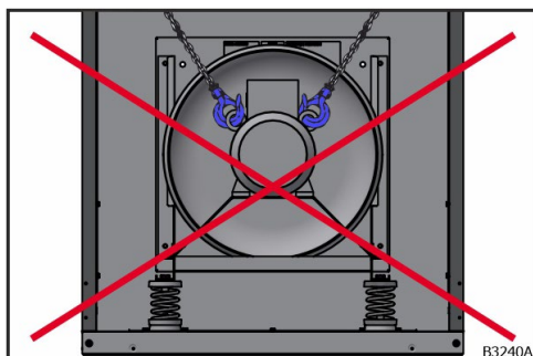
Obr. 33: Nesprávne uviazané bremeno
