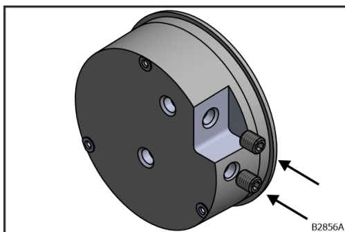
Obr. 131: Zatvorenie so závitovými kolíkmi
