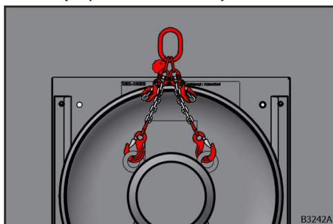
Obr. 81: Zavesenie viazacích reťazí pri dvoch viazacích ôkoch
