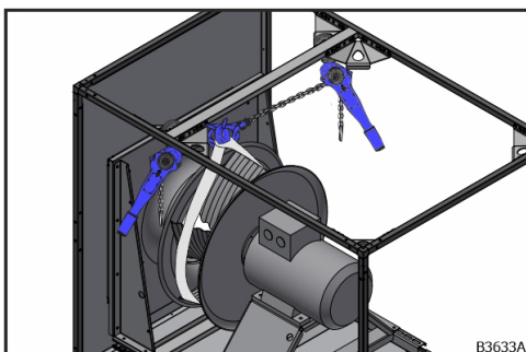
Obr. 44: Pákové reťazové kladkostroje v rohových uzloch
