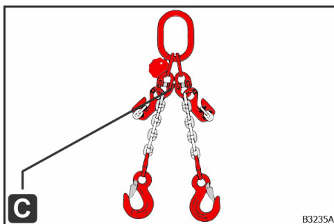
Obr. 28: C – Viazacia reťaz
