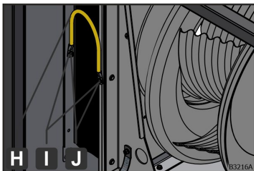
Obr. 21: Kábel na vyrovnanie potenciálov pre pružné napojenie
