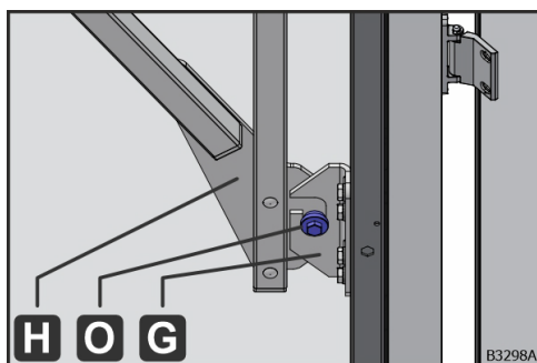
Obr. 111: Centrovacie čapy (O) v závesných uholníkoch dole (G)
