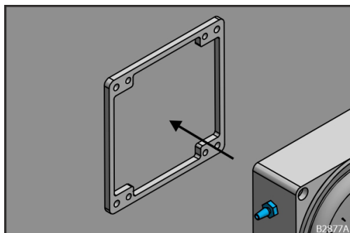
Obr. 154: Umiestnenie opláštenia
