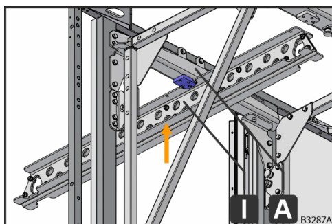
Obr. 67: Zdvihnutie nosného ramena (I) do prednej vodiacej platne
