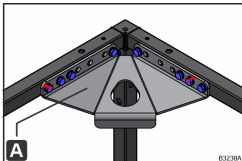
Obr. 51: Pripojenie rohových uzlov
