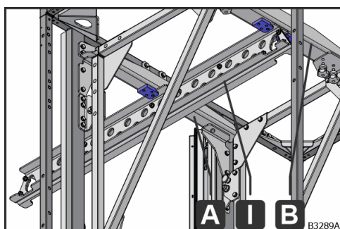
Obr. 69: Zasunutie nosného ramena (I) do zadnej vodiacej platne
