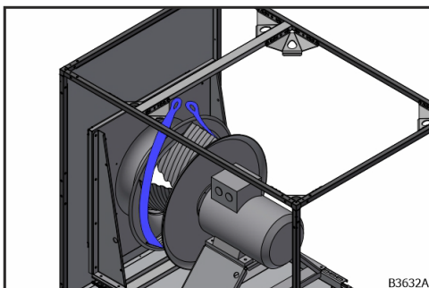
Obr. 43: Obežné koleso s polyesterovou slučkou
