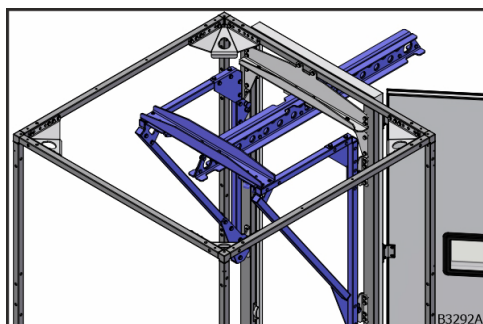
Obr. 72: Hotovo namontovaný vytáhovací modul
