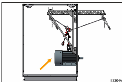
Obr. 102: Bremano v medzistave
