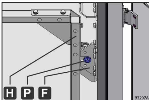
Obr. 75: Centrovacie čapy (P) v závesných uholníkoch hore (F)
