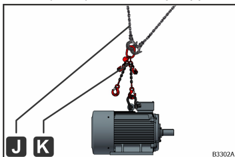
Obr. 100: Závesné háky vo viazacej reťazi (K)
