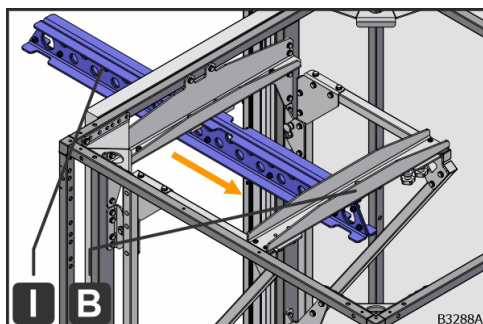
Obr. 68: Zasunutie nosného ramena (I)
