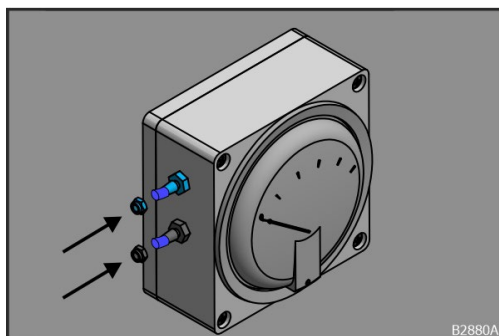
Obr. 158: Naskrutkovanie matíc
