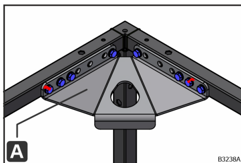
Obr. 30: Pripojenie rohových uzlov
