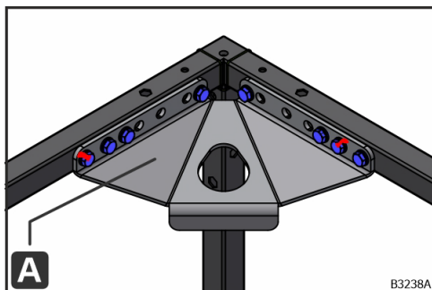
Obr. 73: Pripojenie rohových uzlov
