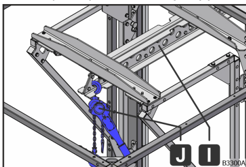
Obr. 98: Vnútorňý viazací bod
