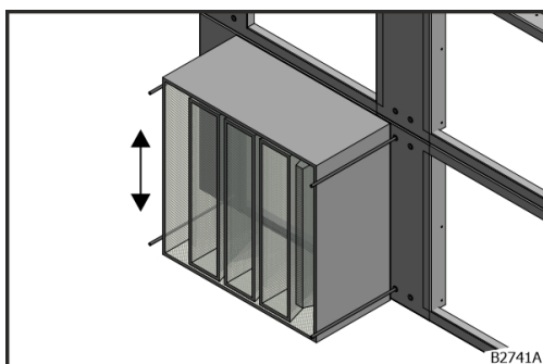
Obr. 13: Vyrovnávanie filtra
