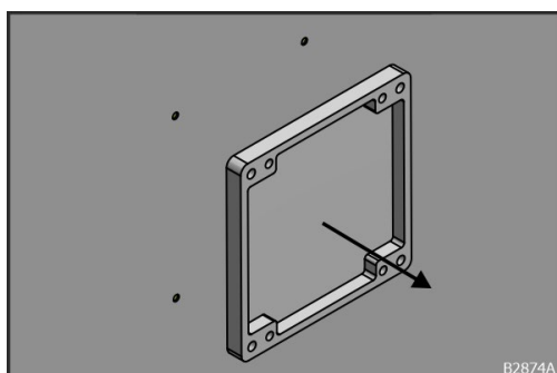
Obr. 148: Odobratie opláštenia
