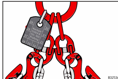
Obr. 50: Kontrolná značka (viazacia reťaz)
