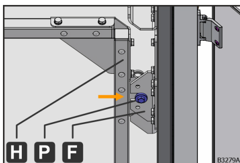
Obr. 60: Zavedenie centrovacieho čapu hore do drážky
