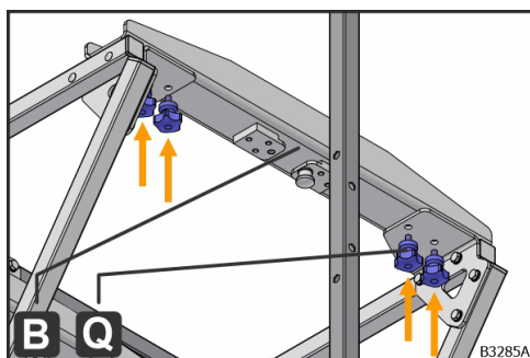
Obr. 65: Zaskrutkovanie pripojovacieho profilu (B)
