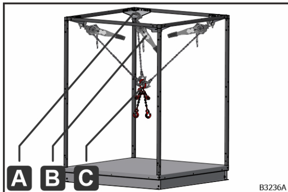
Obr. 24: Konštrukcia prípravku na vyberanie motora
