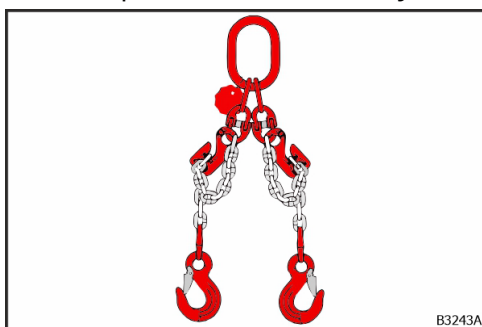
Obr. 34: Použitie reťazových skracovacích hákov
