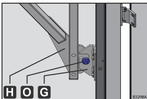
Obr. 76: Centrovacie čapy (O) v závesných uholníkoch dole (G)
