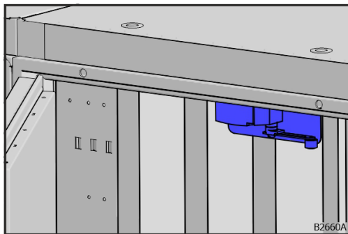
Obr. 119: Kontaktný spínač dverí
