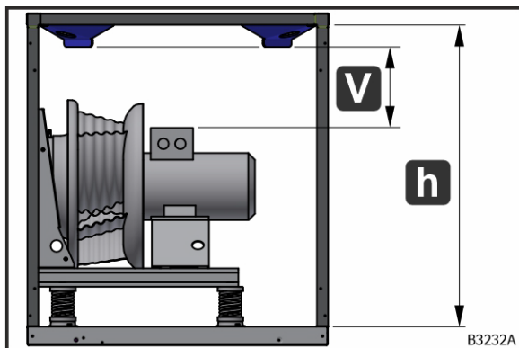
Obr. 25: Minimálna vzdialenosť (V) medzi rohovými uzlami a bremenom.
