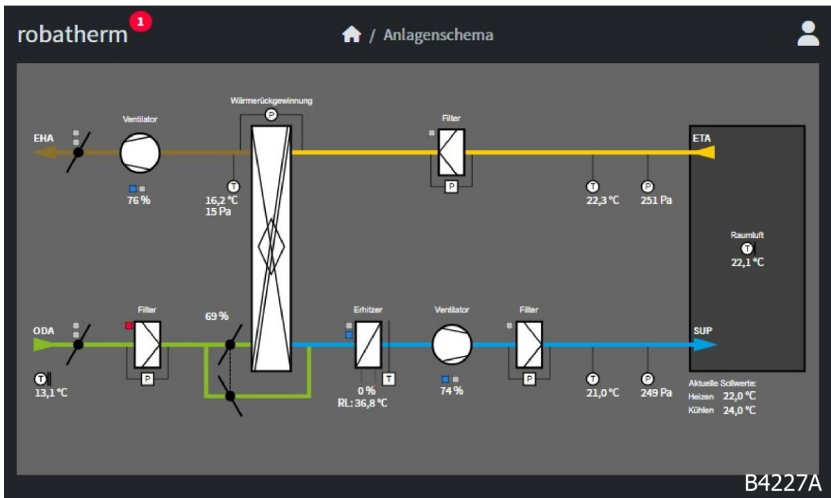
Abb. 19: Beispiel Anlagenschema
