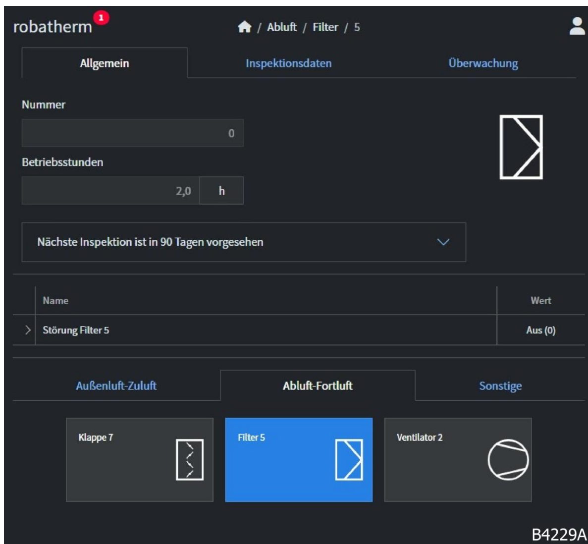
Abb. 18: Beispiel Detailseite Filtereinheit
